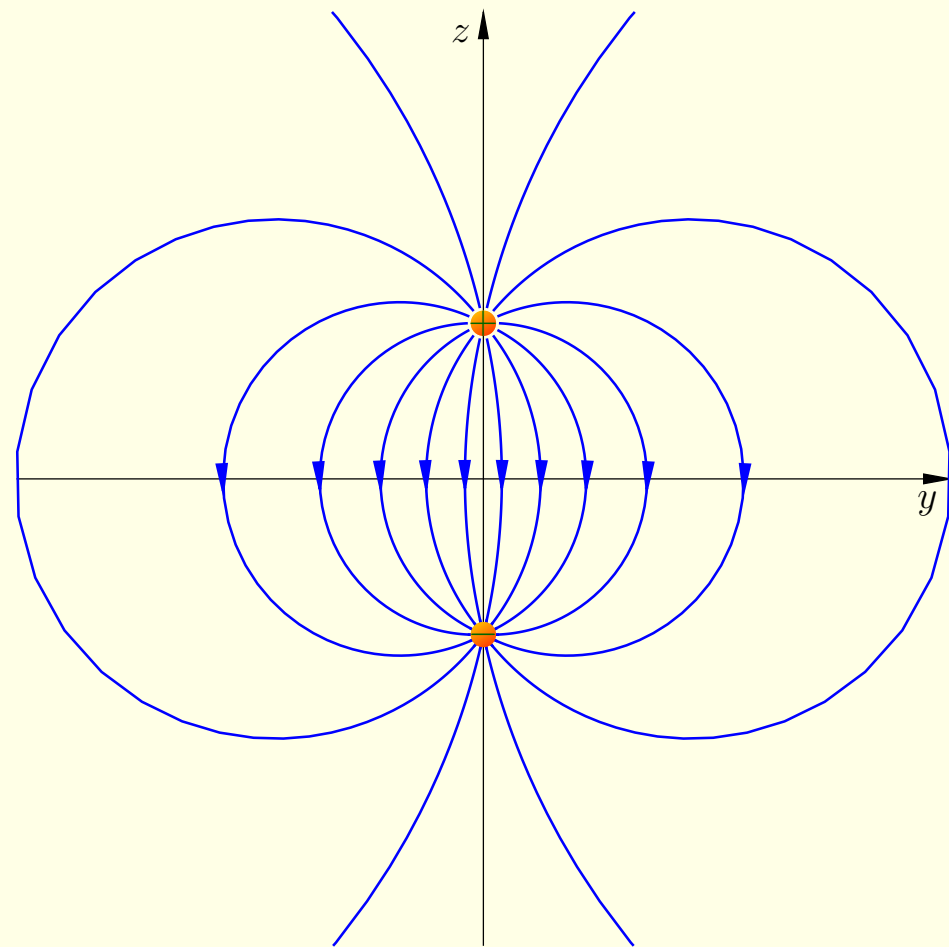
pole dipola fizycznego
