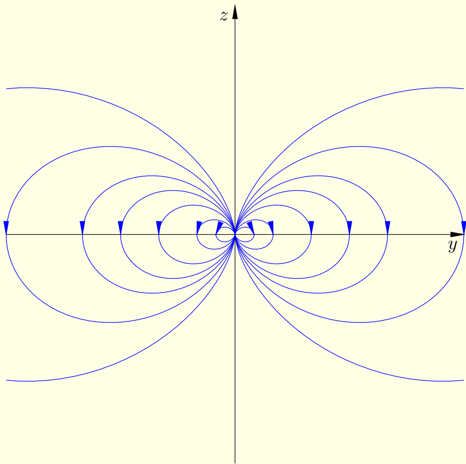
pole „idealnego” dipola
